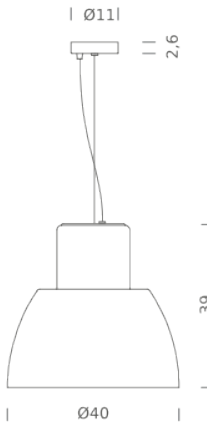
LOROSAE Ø40
